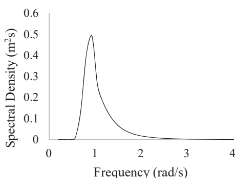
Fig. 3 JONSWAP Spectrum
