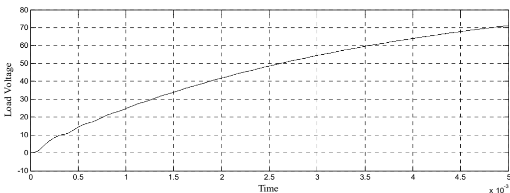
Fig. 12 Load voltage
