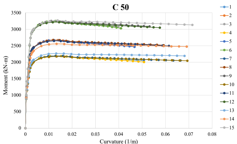
Fig. 5 (d) MC relationship for C50
