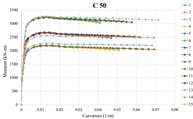
Fig. 5 (d) MC relationship for C50
