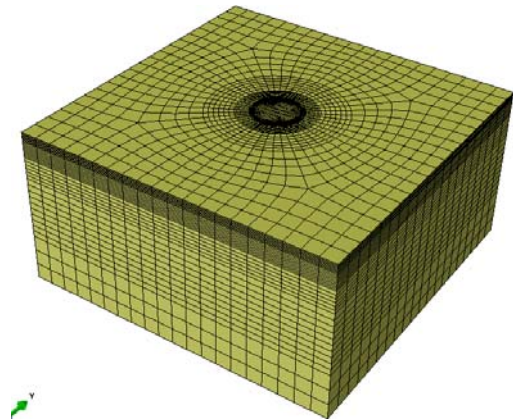
Fig. 2 FEM Mesh
